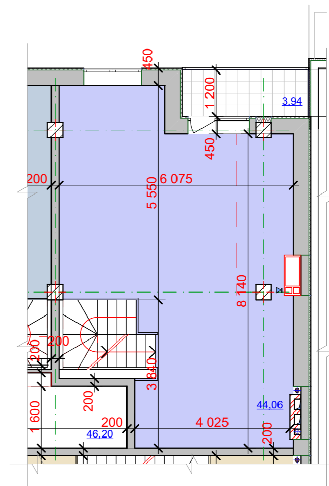
третій поверх 3х рівневої квартири 1А Секція 7, поверх 11й
