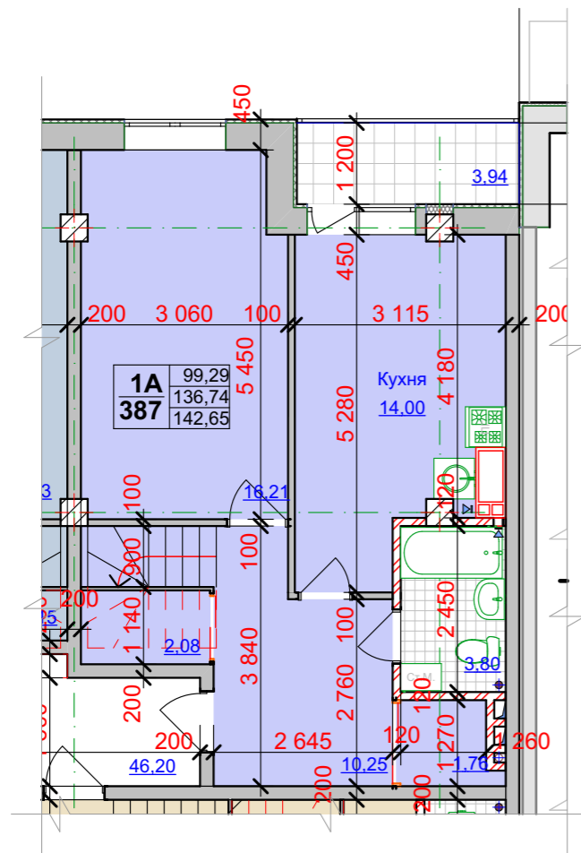
перший поверх 3х рівневої квартири 1А Секція 7, поверх 9й
