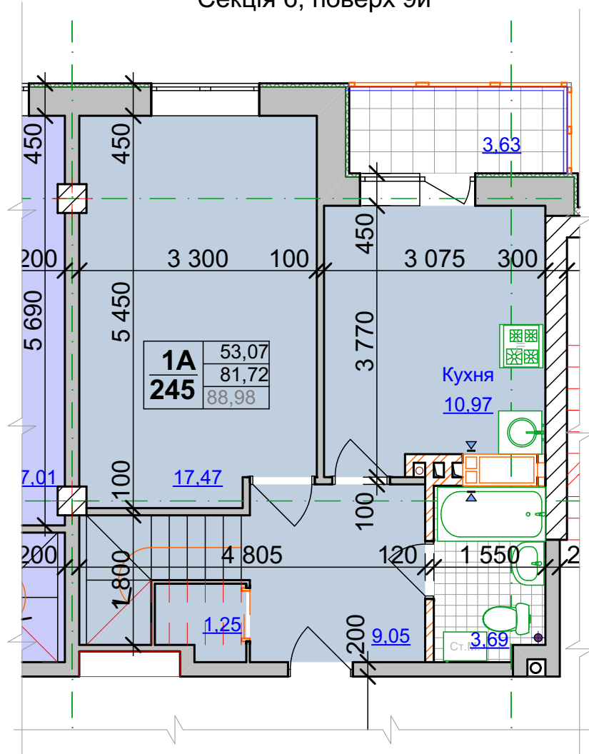
перший поверх 2х рівневої квартири 1А Секція 6, поверх 9й
