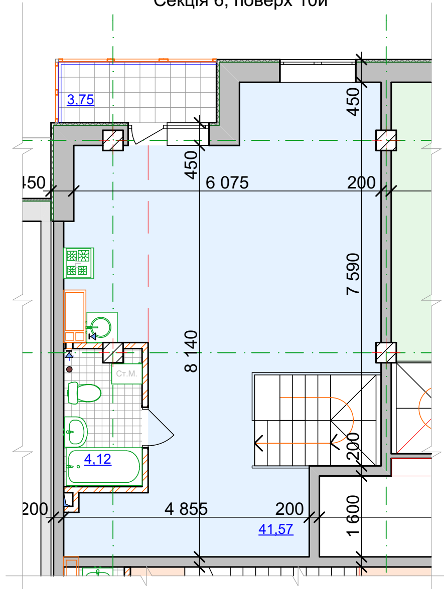
другий поверх 2х рівневої квартири 1Б Секція 6, поверх 10й
