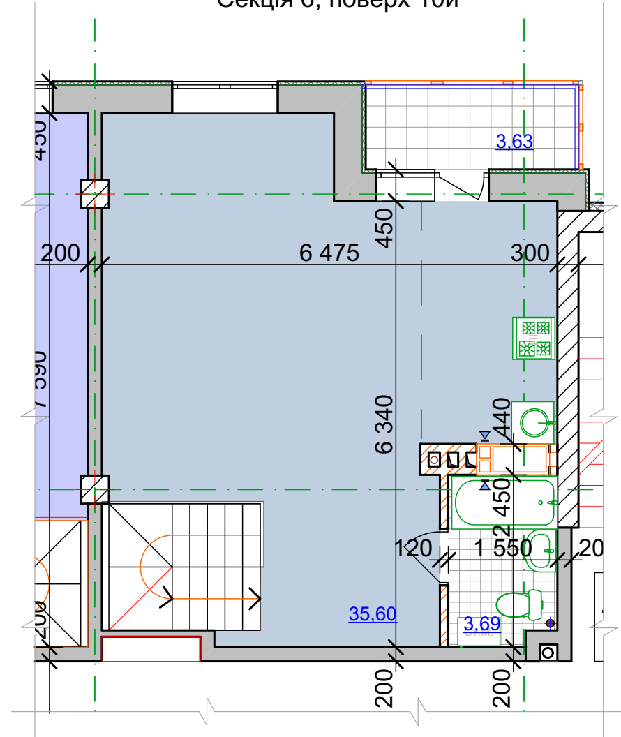
другий поверх 2х рівневої квартири 1А Секція 6, поверх 10й
