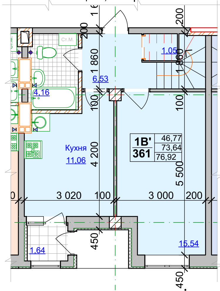
перший поверх 2х рівневої квартири 1В' Секція 6, поверх 9й
