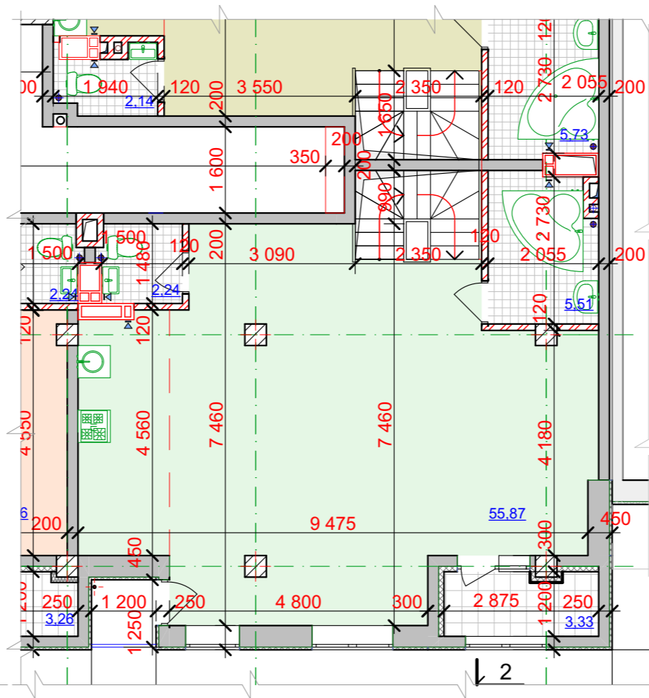
другий поверх 3х рівневої квартири 2В Секція 5, поверх 10й
