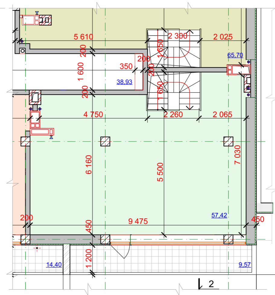
третій поверх 3х рівневої квартири 2В Секція 5, поверх 11й
