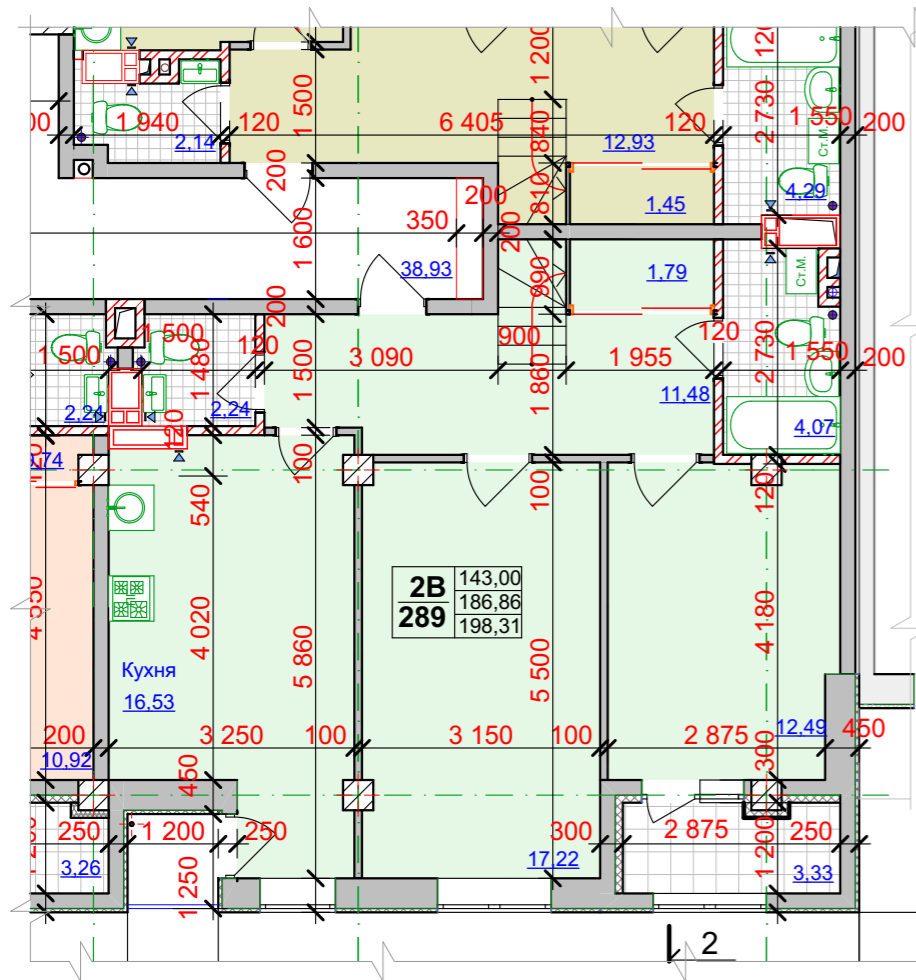
перший поверх 3х рівневої квартири 2В Секція 5, поверх 9й
