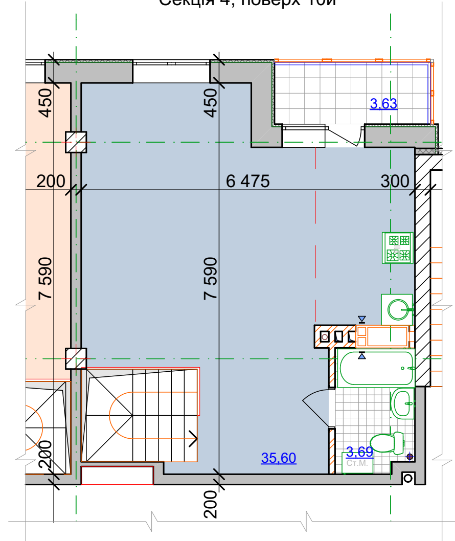
другий поверх 2х рівневої квартири 1А Секція 4, поверх 10й
