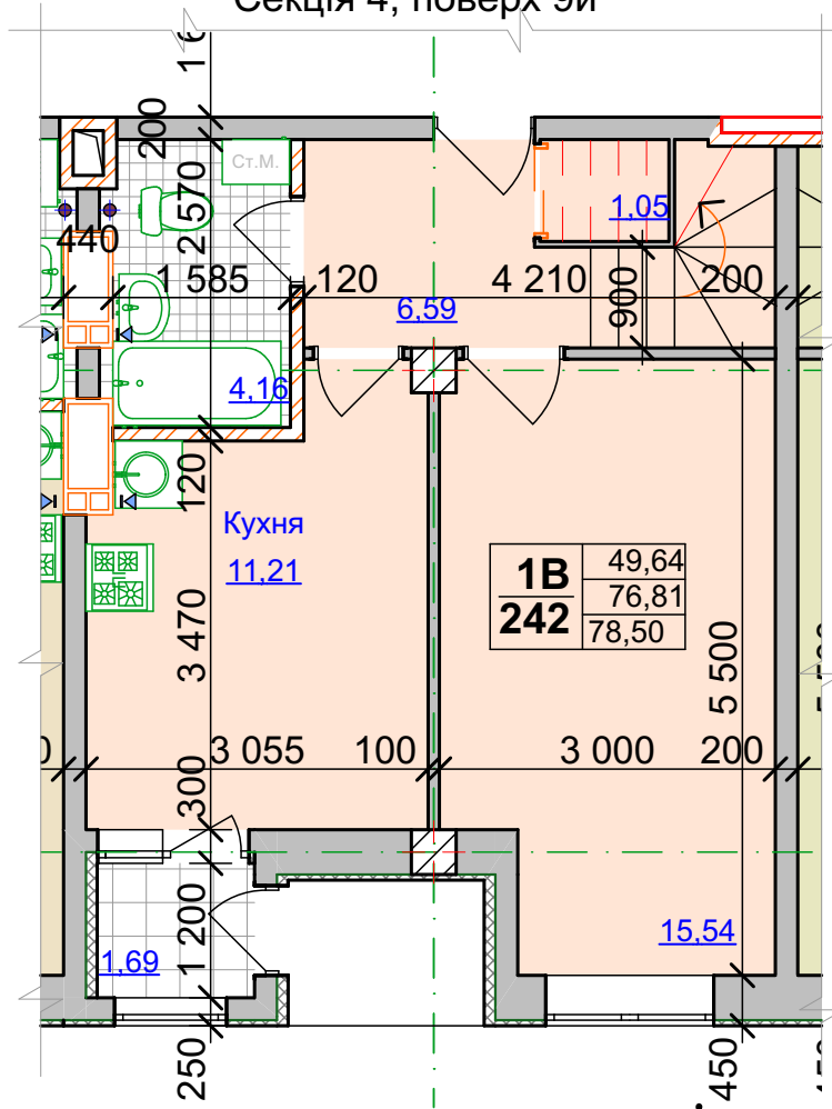
перший поверх 2х рівневої квартири 1В Секція 4, поверх 9й
