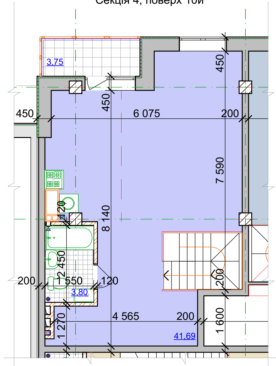
другий поверх 2х рівневої квартири 1Б Секція 4, поверх 10й
